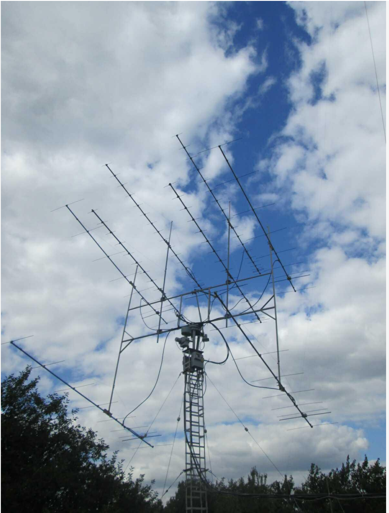
UXoFF antenna: 144 MHz 4x9 ; 432 MHz 4x19.
